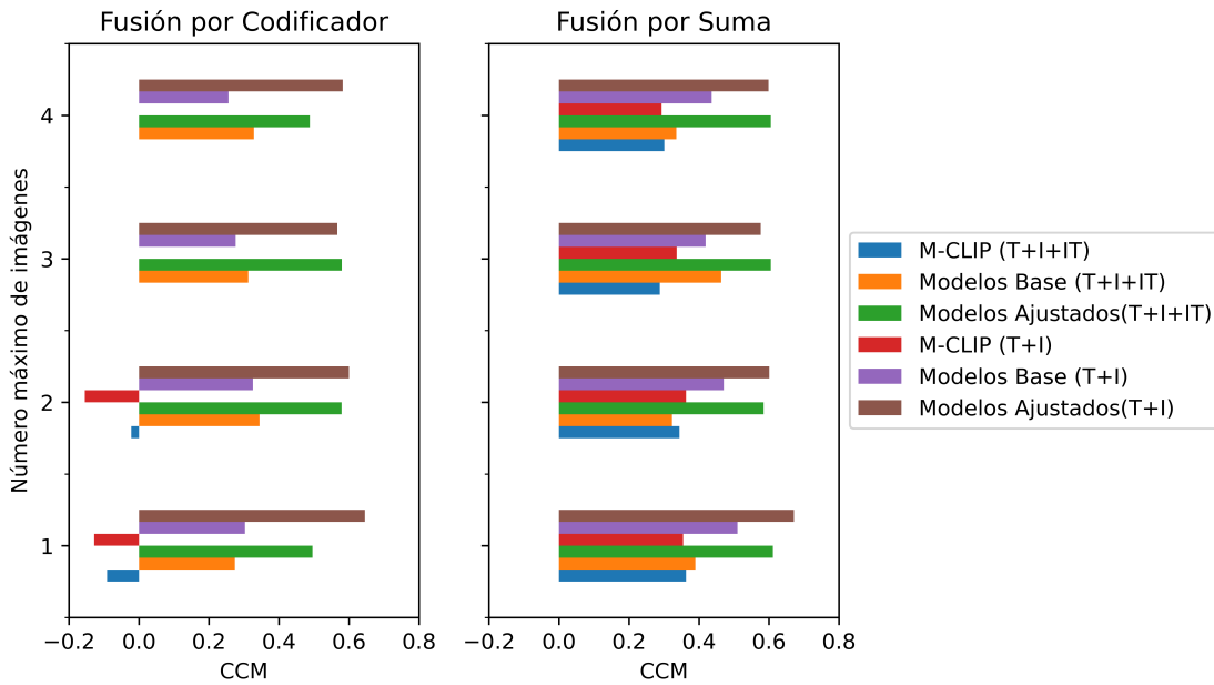
FIGURA 4.14: Puntuaciones según el CCM para los distintos modelos de clasificación, los dos modos de fusión de información, y diferentes tipos de información, cambiando el número máximo de imágenes que se agregan a ellos. Fuente: elaboración propia.
