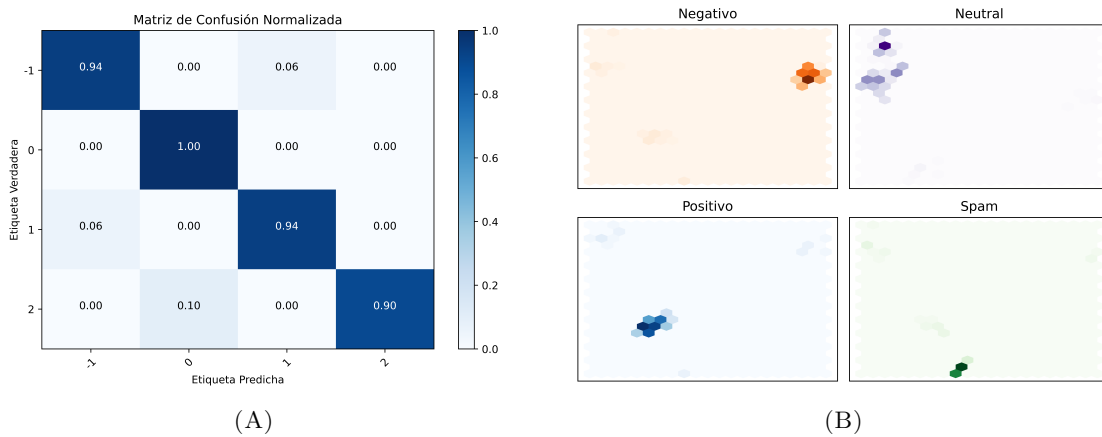
FIGURA 4.19: (A) Matriz de confusión y (B) proyecciones 2D de los embeddings del mejor modelo obtenido: 96.00% CCM para tuits fusionados por fusión por suma, BETO y ViT ajustados, texto e imágenes, considerando únicamente las primeras tres imágenes de cada publicación. Fuente: elaboración propia.
