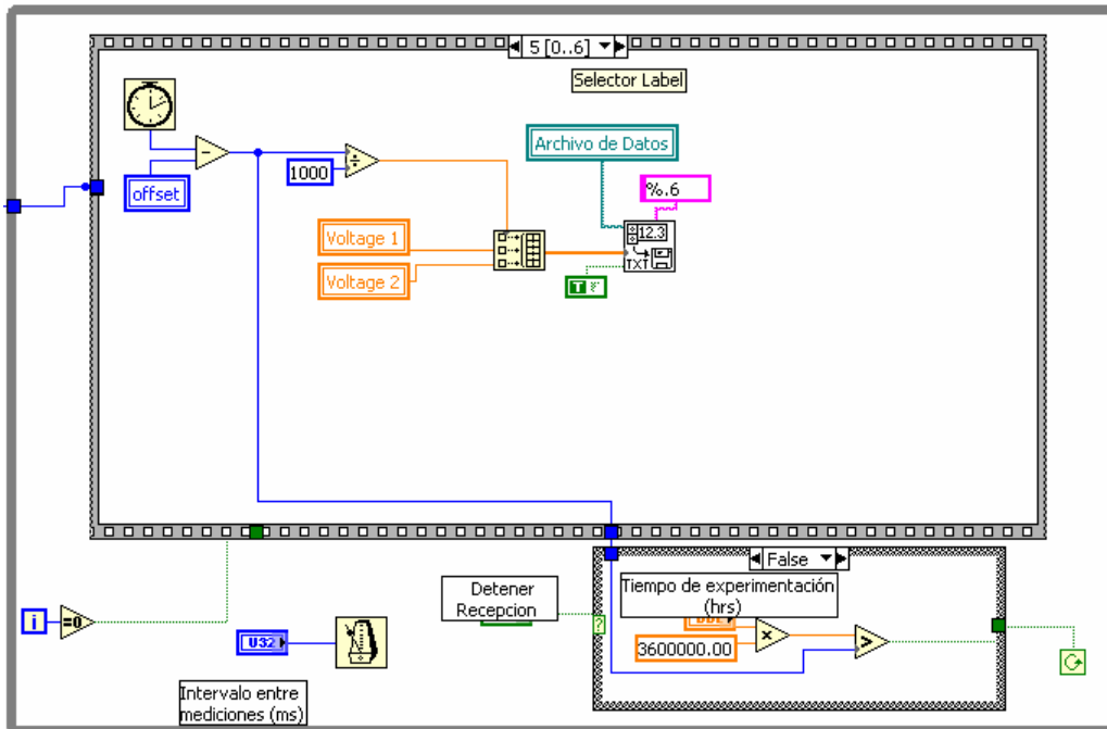
Figura A 3.2 Programa LabVIEW, diagrama correspondiente a la parte de recolección y almacenamiento de datos
