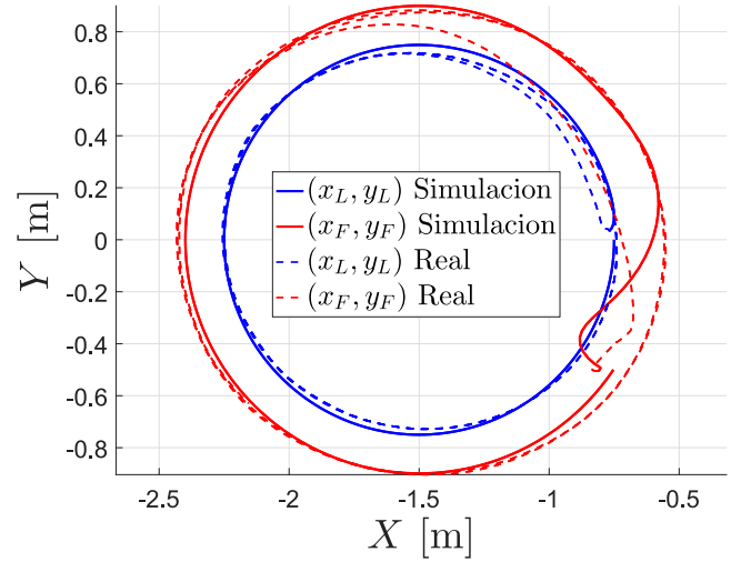
Figura 3. Trayectoria en el plano.
