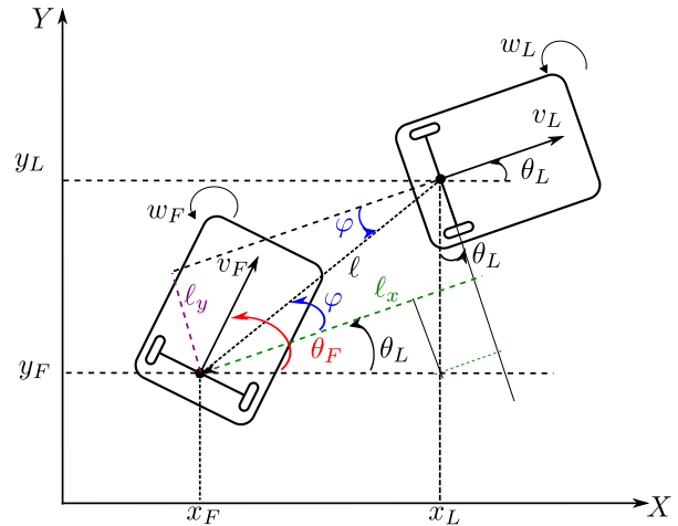
Figura 1. Esquema líder-seguidor.
