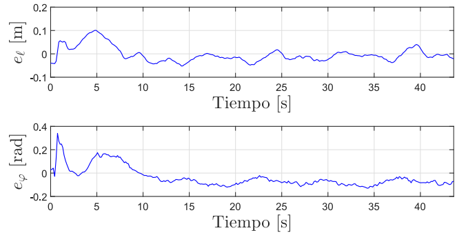
Figura 4. Errores de distancia y ángulo.
