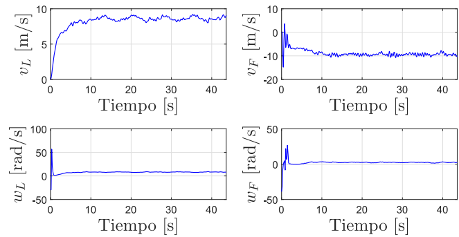
Figura 5. Entradas de control.
