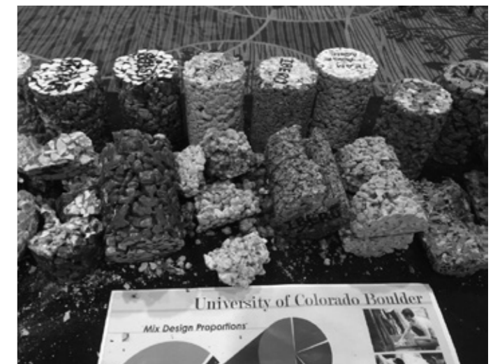
Competencia sobre diseño de concreto permeable. Convención Otoño 2015 del American Concrete Institute (ACI). Denver, Estados Unidos. Especímenes de prueba.
