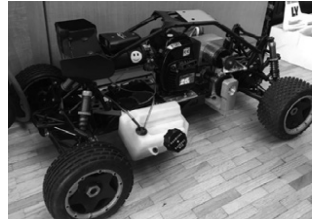
Prototipo Funcional del VEH a escala.
