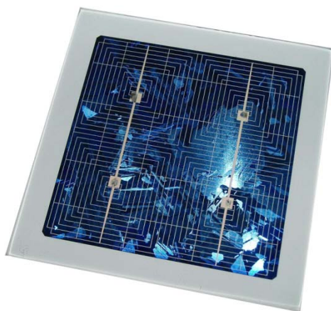
Celda fotovoltaica policristalina solar de 4 pulgadas
